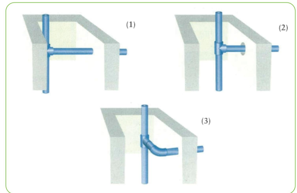
Hình 4. Lắp ớng trong trục Figure 4. Installation in vertical pipe
