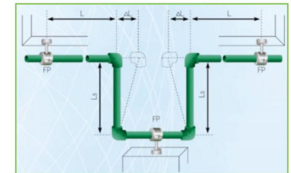
Hình 2. Vòng giãn nở Figure 2. Expansion ring
