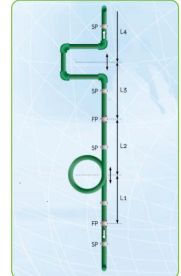
Ví dụ về bù giãn nở trong đoạn thẳng của ống bằng uốn tròn và loại U (Example of linear expansion compensation in a straight section of pipe circle bend and U-type compensator)
