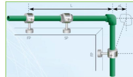
Hình 1. Nhánh giãn nở Figure 1. Expansion Branch
