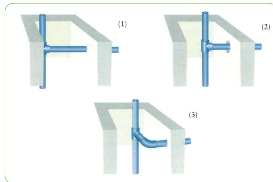
Hình 4. Lắp ống trong trục Figure 4. Installation in vertical pipe
